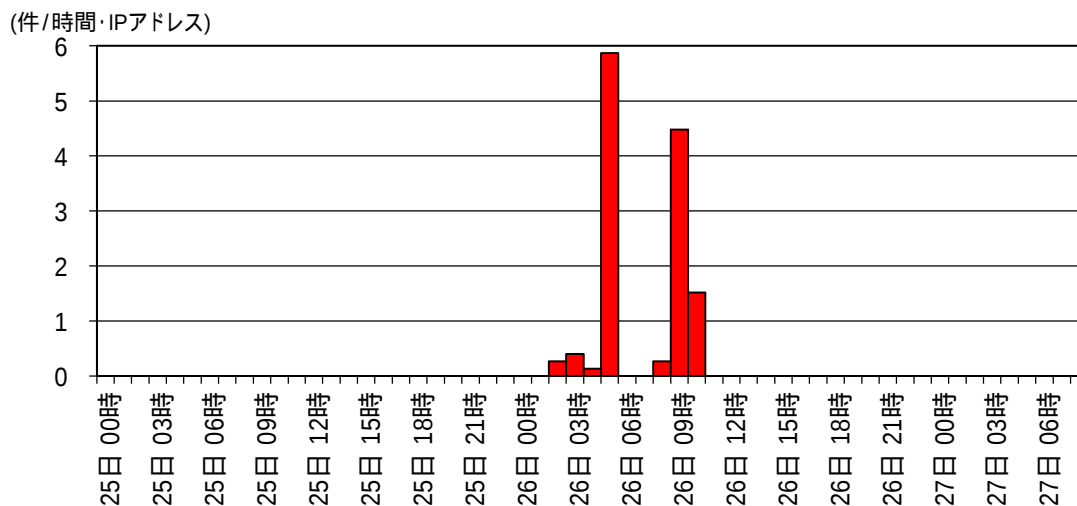
図1 Apache Struts2 の脆弱性を狙ったアクセスの検知状況 (H26.4.25 00:00 ~ H26.4.27 08:59)
