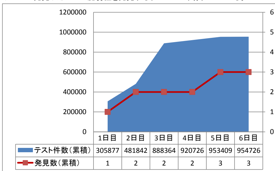
図 31 ブロードバンドルータ D におけるファジングのテスト件数と脆弱性発見数
