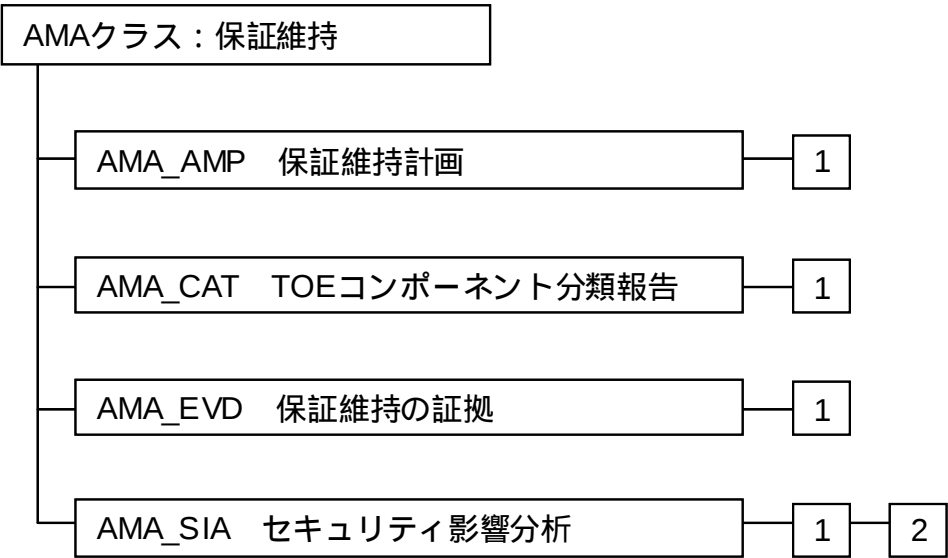
図 16.1 - 保証維持クラスのコンポーネント構成
