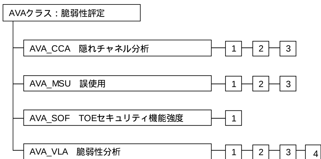
図 14.1 - 脆弱性評価クラスのコンポーネント構成
