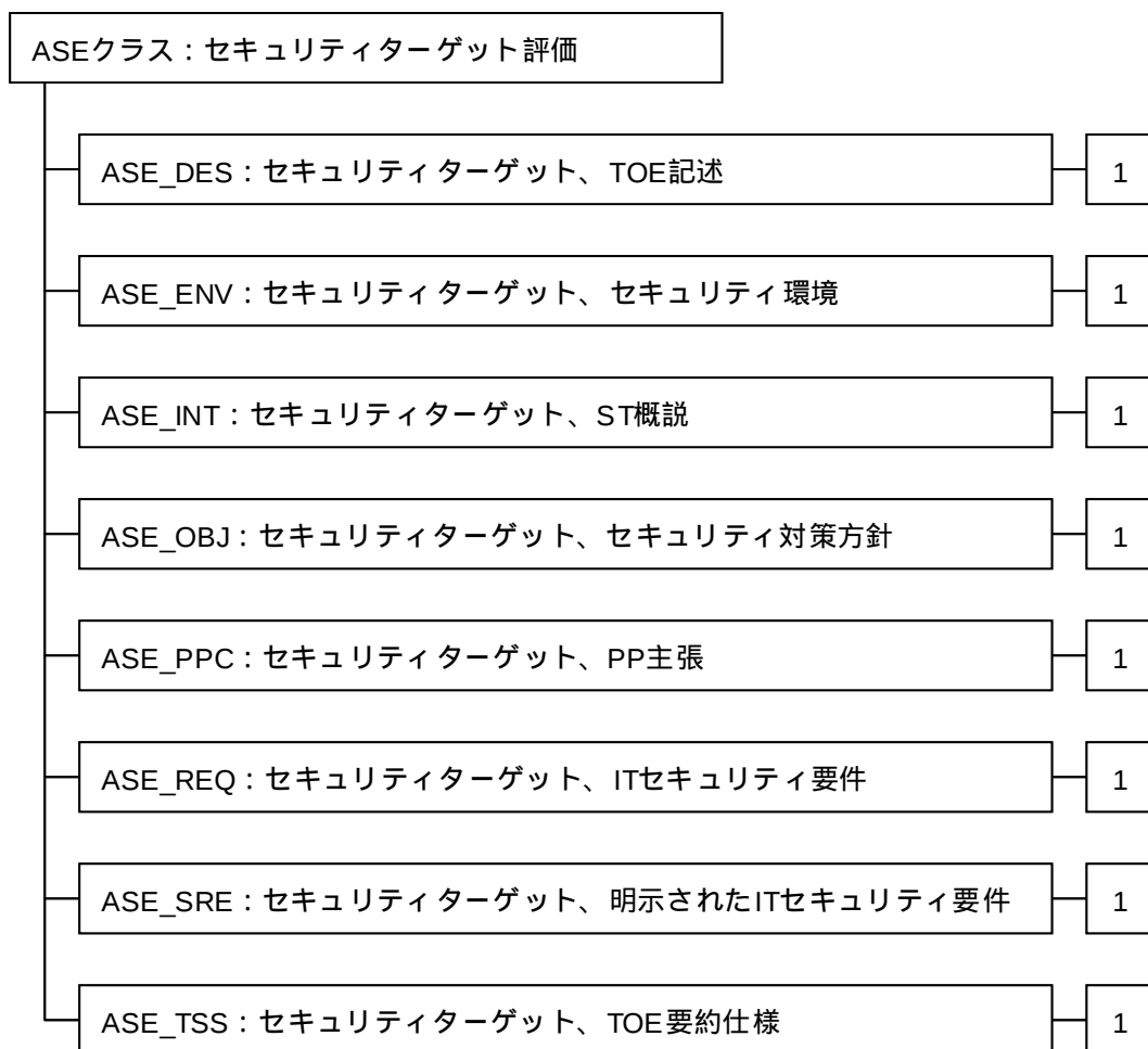
図 5.1 - セキュリティターゲット評価クラスのコンポーネント構成
