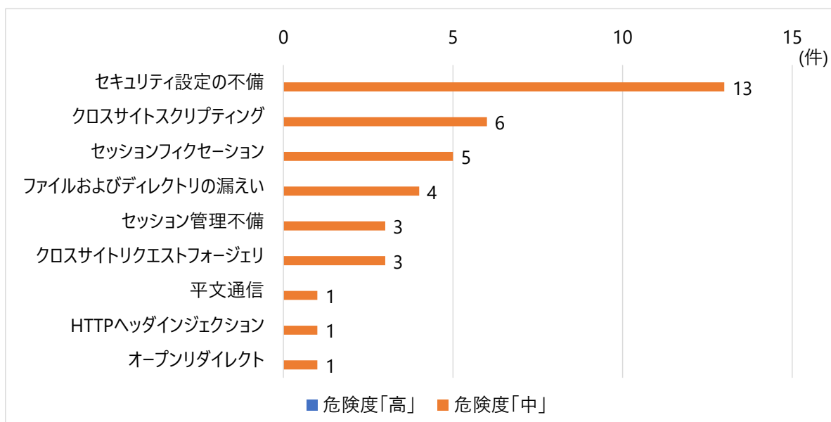
Web アプリケーション診断における延べ検出数上位の脆弱性カテゴリ (診断事業者 A が実施した診断対象企業 20 社の集計結果)
