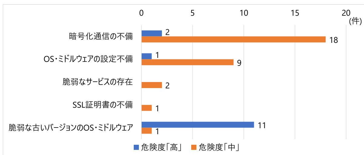
プラットフォーム診断における延べ検出数上位の脆弱性カテゴリ (診断事業者 B が実施した診断対象企業 30 社の集計結果)
