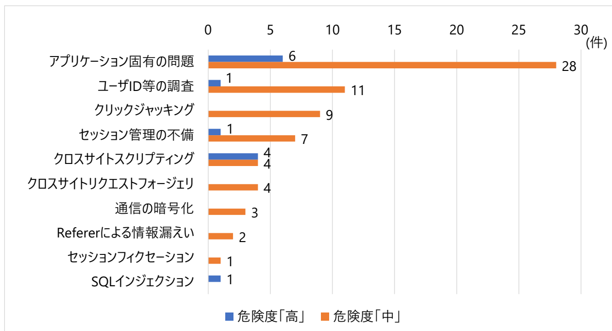
Web アプリケーション診断における延べ検出数上位の脆弱性カテゴリ (診断事業者 B が実施した診断対象企業 30 社の集計結果)
