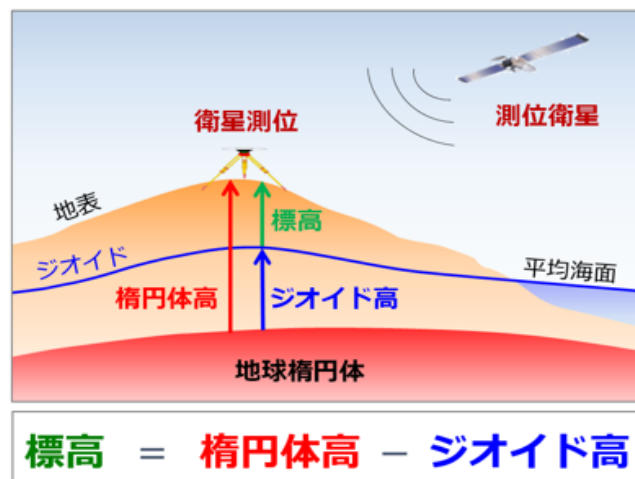
図 2-5 楕円体高、ジオイド高、標高の関係 2 （一部離島を除く 3 ）
