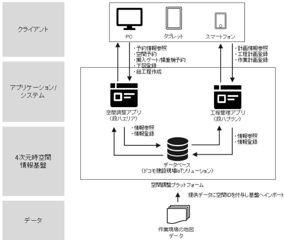
図 3-3-2 システムアーキテクチャ
